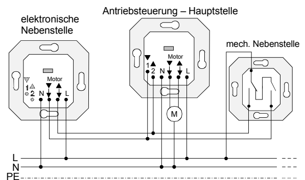
Bild: Jalousiesteuerungseinsatz „Universal“ mit mechanischer und elektronischer Nebenstelle
