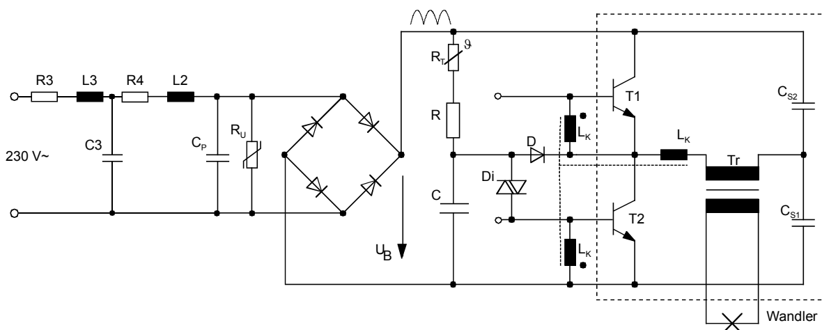
Bild: Grundschialtung TRONIC-Trafo
