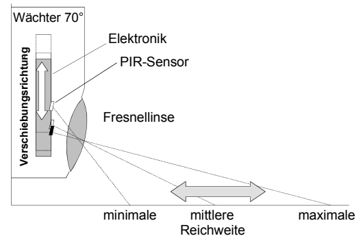
Bild: Reichweitenverstellung beim Wächter 70
