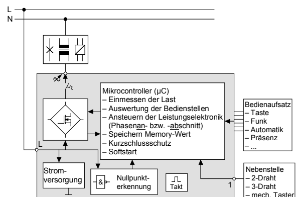
Bild: „System 2000“-Universal-Dimmeinsatz – Blockschaltbild
