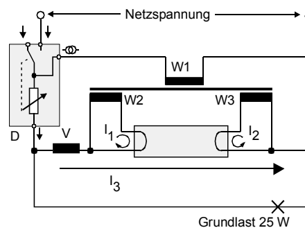
Bild: Leuchtstofflampe mit Heiztrafo und Dimmer
