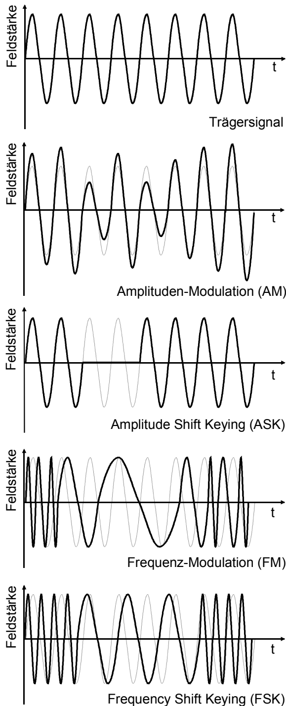
Bild: Modulationsarten
