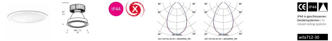
Downlight mit Streuscheibe, 3000 K / Downlight with Diffusing screen, 3000 K
