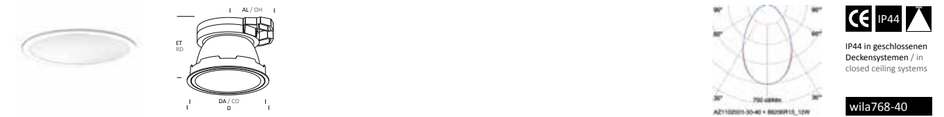
Downlight mit Streuscheibe, 4000 K / Downlight with Diffusing screen, 4000 K
