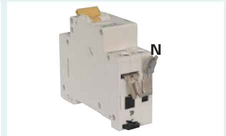
Gleicher Anschlusswinkel ZV-N-05TE für Polstreife N (CLS6 mit 1,5TE) 50 und 80 A Verschiebung
