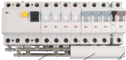
Sammelschiene ZV-SS ZV-SS-80A Abdeckprofil ZV-ADP Endkappen ZV-AEK
