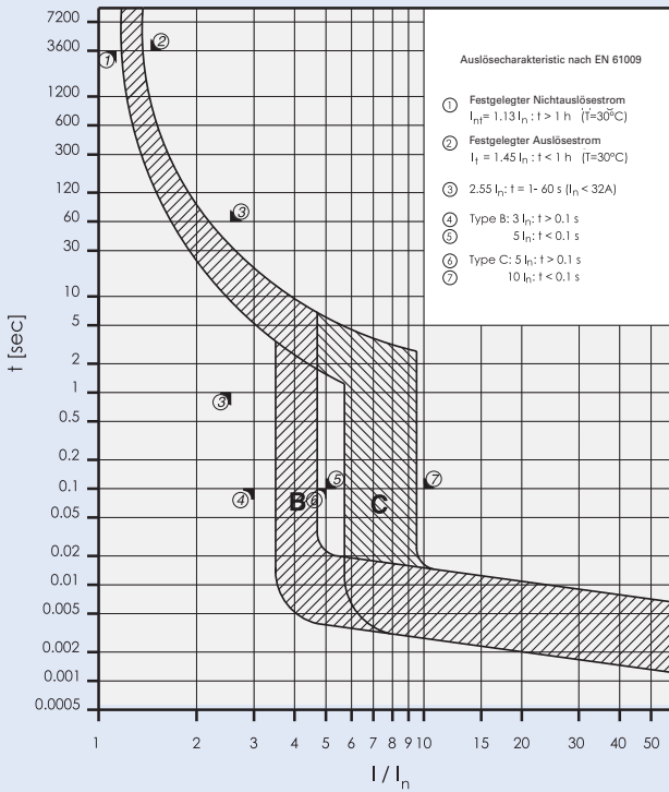
Auslösecharakteristik AFDD+, Kennlinien B und C
