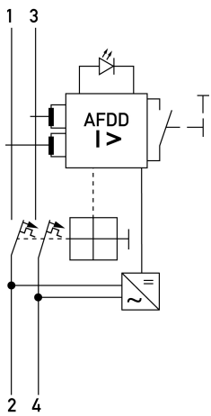
Anschlusschema
