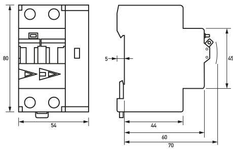
Maßzeichnung Gruppenansicht
